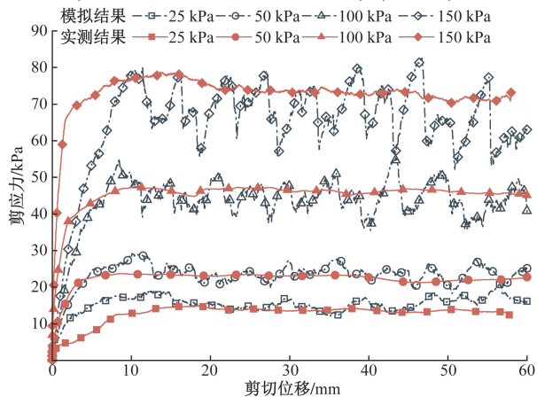
图 5 直剪试验与离散元模拟试验结果 Fig. 5 Results of direct shear test and discrete element simulation test
