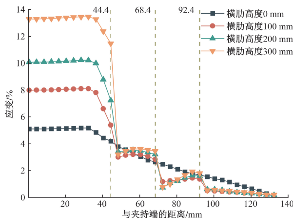
图 16 不同横肋高度的水平土工织物应变曲线 Fig. 16 Strain curves of horizontal geotextiles with different rib heights
