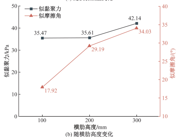
图 12 界面强度参数变化曲线
