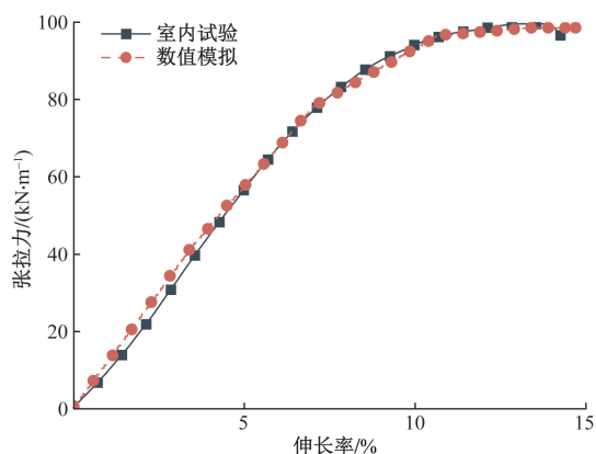
图 2 土工织物拉伸曲线实测值与模拟值对比
