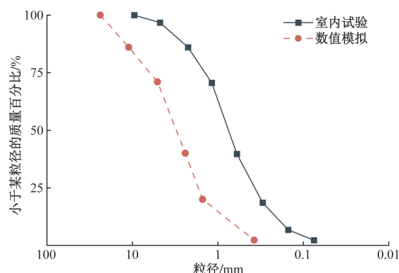
图 4 室内试验与离散元模型的颗粒级配曲线
