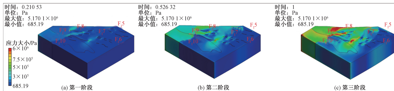
图 13 第三期模拟等效应力分布图
