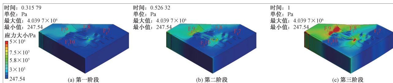
图 12 第二期模拟等效应力分布图
