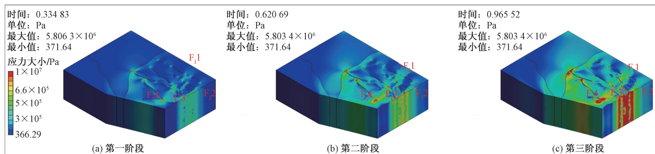
图 11 第一期模拟等效应力分布图
